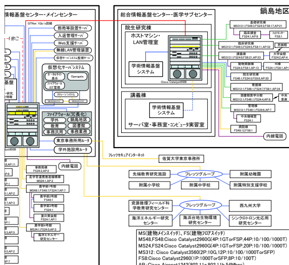
質大学キャンパス情報ネットワークシステム構成図
