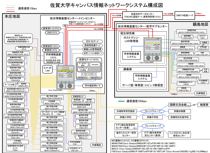
図 4.7: キャンパス情報ネットワークシステム構成
