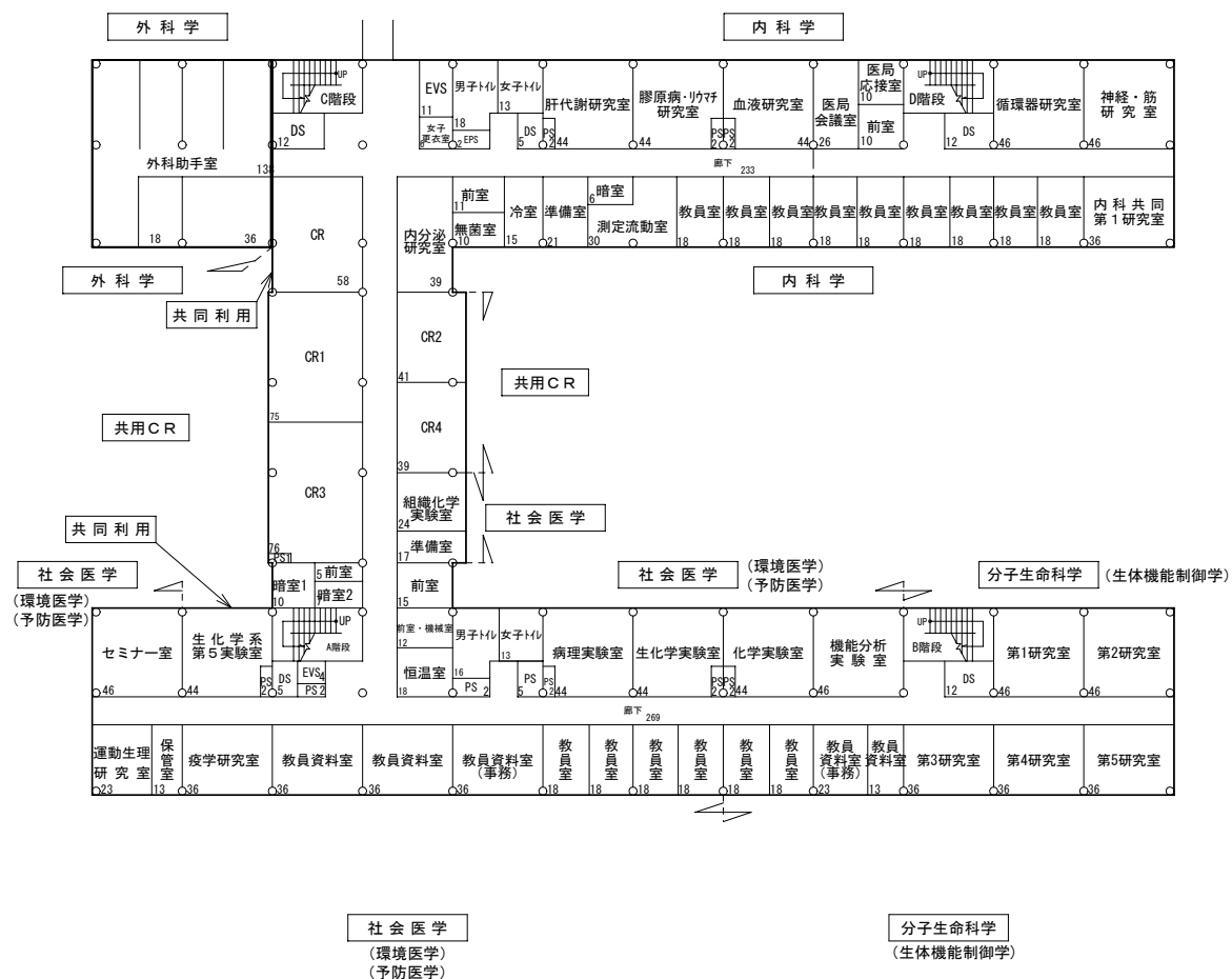
4 階 平 面 図 S=1/600
