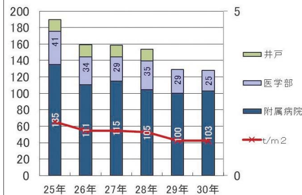
図3 水使用量(千m 3 )
