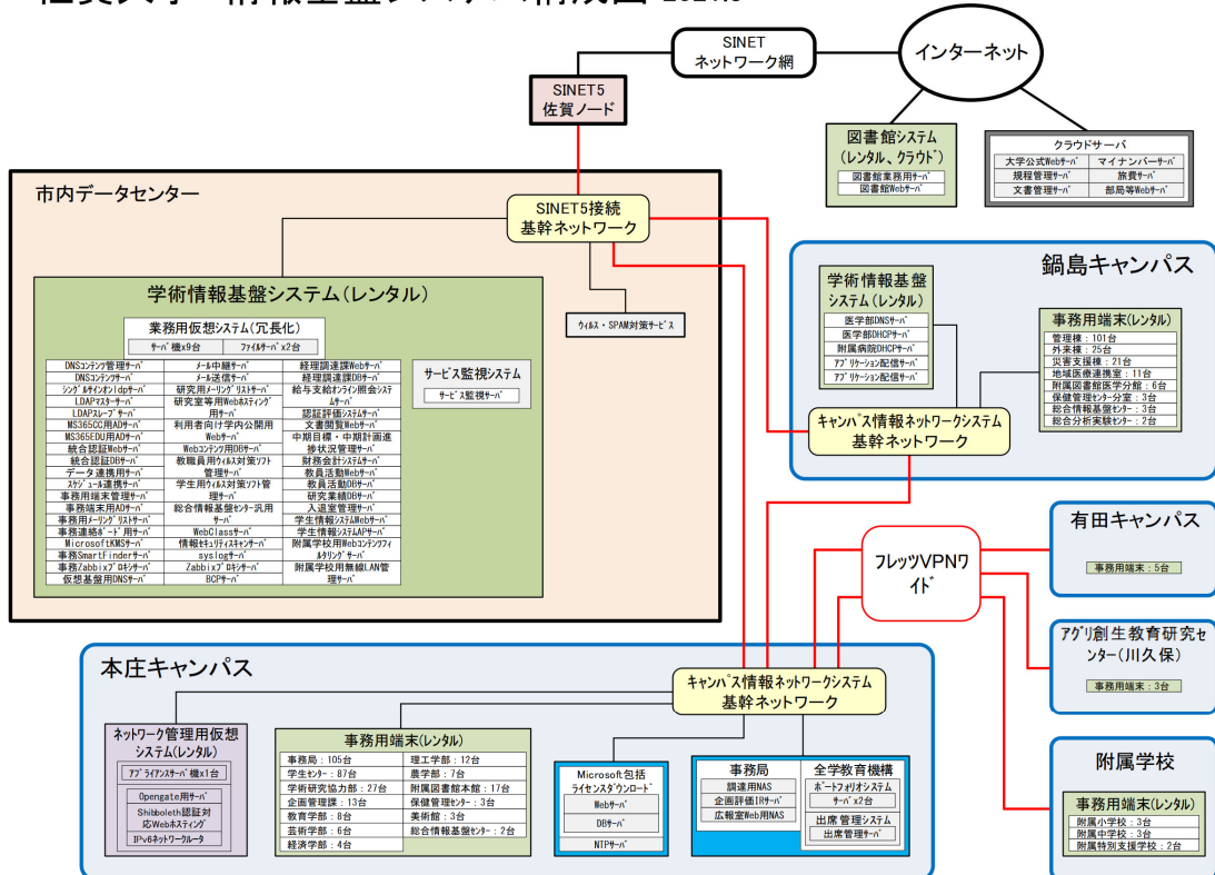
図 4.1 佐賀大学情報基盤システム構成図（2021年3月）
