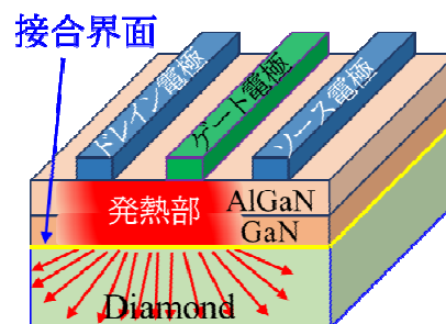
高放熱性GaNトランジスタ
